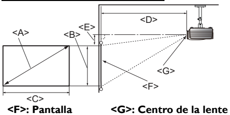
Instalación en el techo
