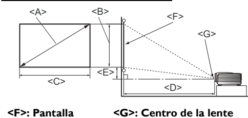
Instalación en el suelo
